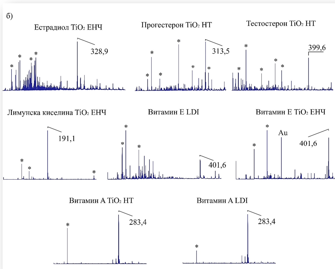
Слика 3.17. б) SALDI TOF масени спектри детектованих негативних јона следећих молекула: естрадиол, тестостерон, прогестерон, лимунска киселина, витамин Е и витамин А са једним од нанокристала TiO 2 са којим даје највећи број сигнала чије су S/N вредности анализиране у даљем раду. За витамине су дати и спектри снимљени без матрице ради поређења, на слици су означени као „Витамин Е LDI“ и „Витамин А LDI“.
