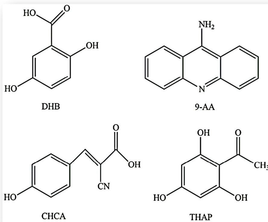
Слика 1.2. Структурне формуле органских матрица: 2,5-дихидроксибензоева киселина, DHB, 9-аминоакридин, 9-AA, α-цијано-4-хидроксициметна киселина, CHCA, 2,4,6-трихидроксиацетофенон, THAP.
