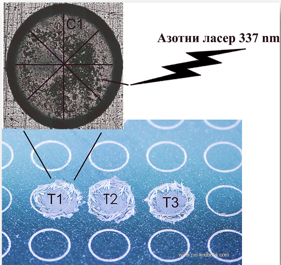
Слика 2.1. Илустрација експеримента за тестирање репродуцибилности и хомогености система. Једно место на MALDI плочи подељено је на осам сектора (C1-C8). Након наношења испитиваних узорака сваки сектор је ексцитован 120 пута ласером (укупно је једно место на плочи ексцитовано 960 пута) и свака комбинација узорка/матрице (или супстрата TiO_2 ) је мерена три пута (T1, T2, T3). Иста процедура је понављана три дана.
