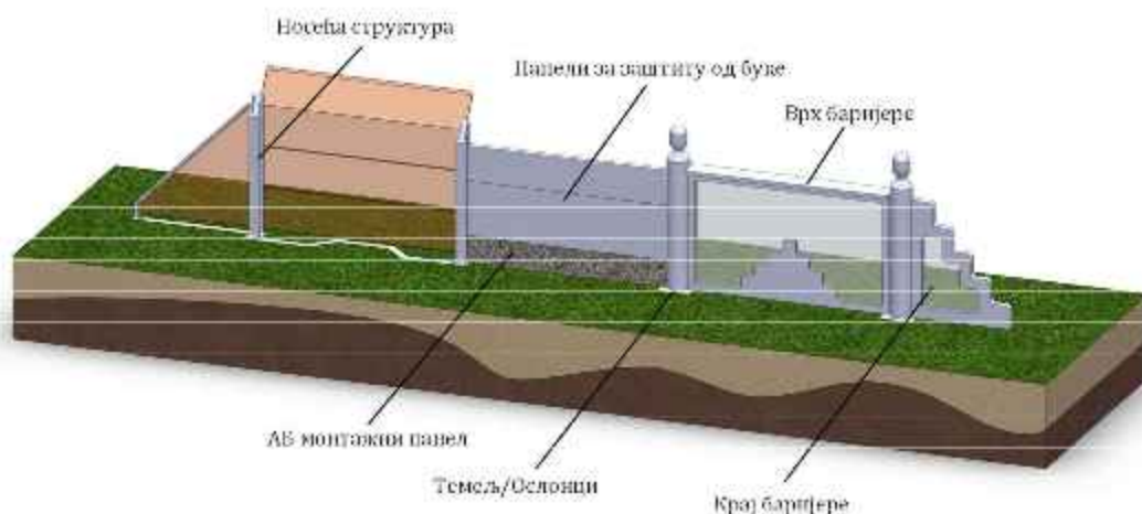
Слика 4.4 Морфологија баријере за заштиту од буке
