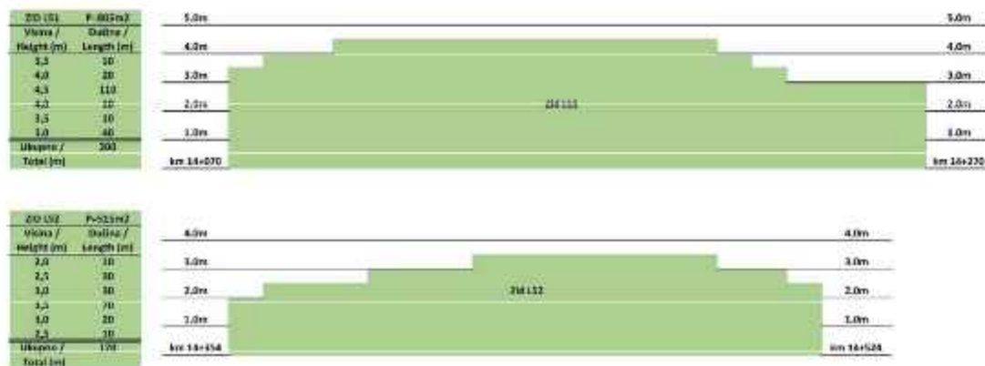
Слика 7.8. Шематски приказ акустичке баријере (Зид L51 и Зид L52) [158]
