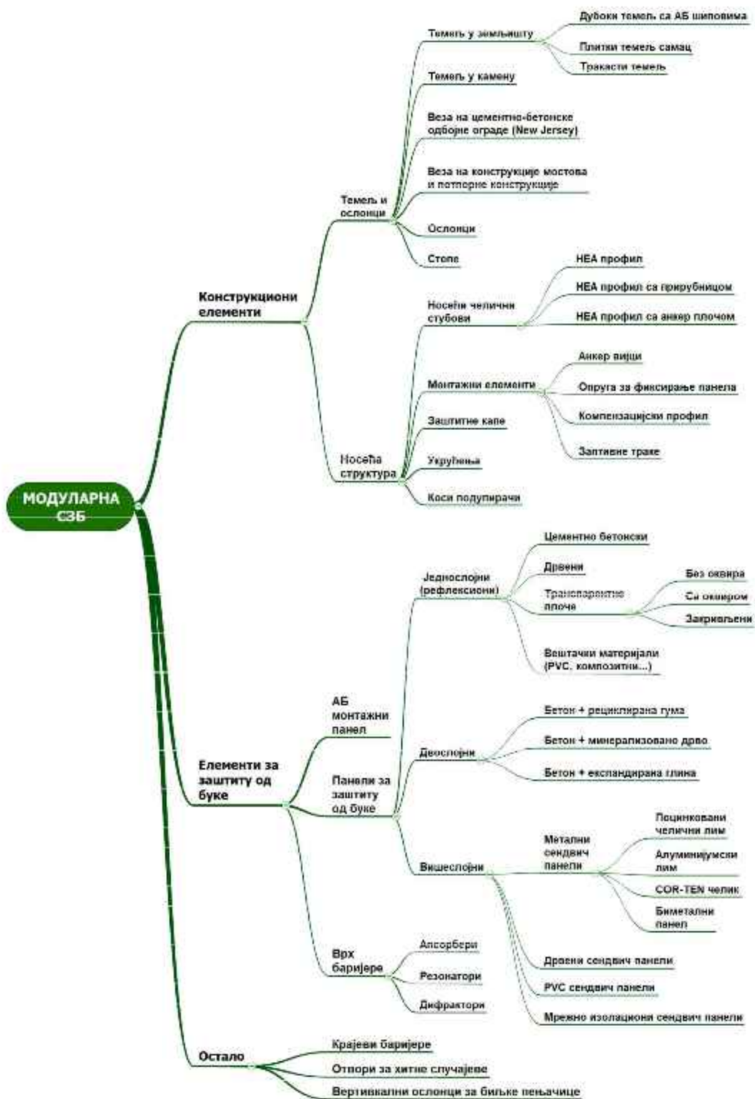
Слика 4.6 Структура модула СЗБ
