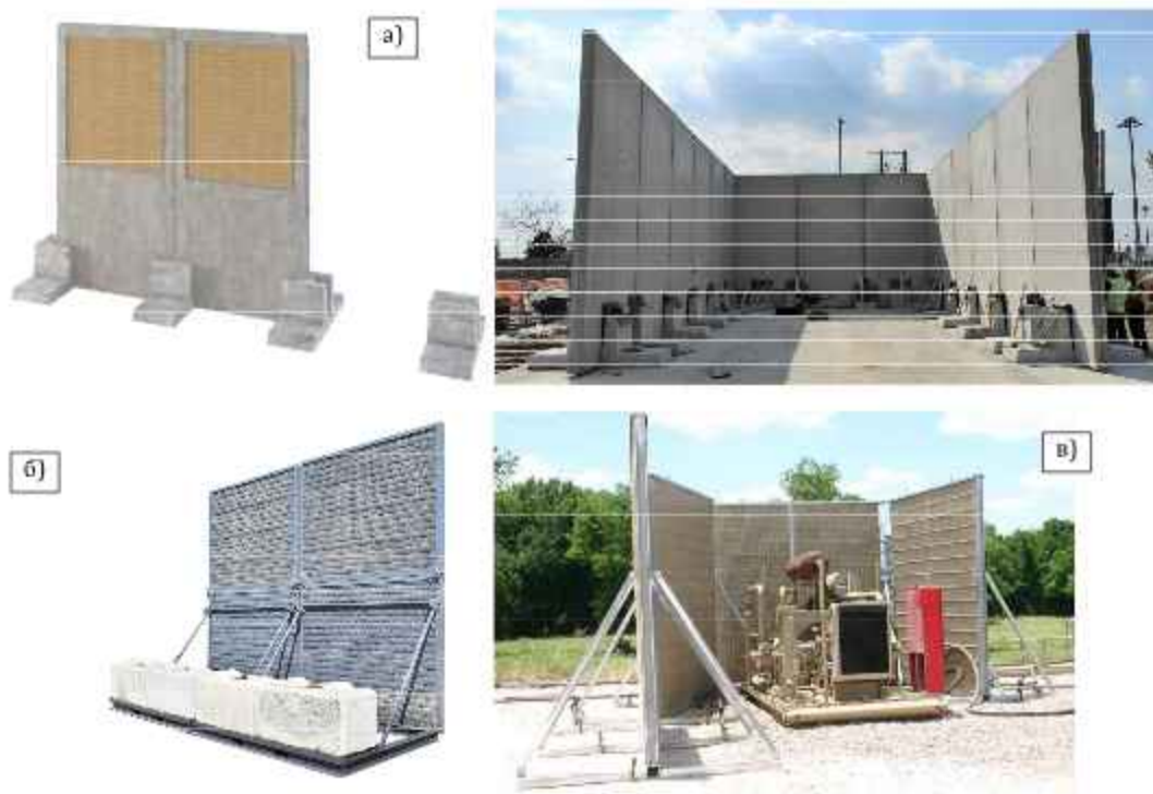
Слика 3.42. Примери самостојећих мобилних баријера са: а) стопама [54], б) ослонцима са контра тежовима [55] и в) косим подупирачима [56]
