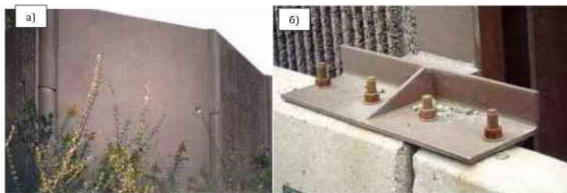
Слика 5.2. Ширење и скупљање материјала: а) везе између панела, б) везе баријера и носећих структура [93]
