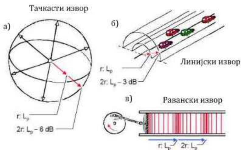
Слика 2.1. Типови извора буке: а) тачкасти извор, б) линијски извор, в) равански извор [21]
