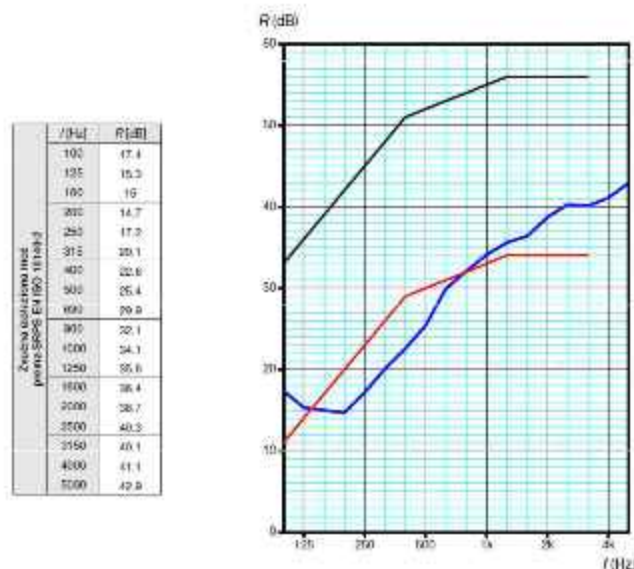
Слика 5.27. Резултати испитивања индекса редукције звука R_i
