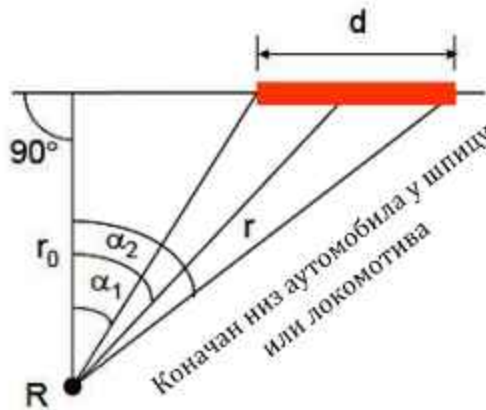
Слика 2.3. Континуални линијски извор буке [1]
