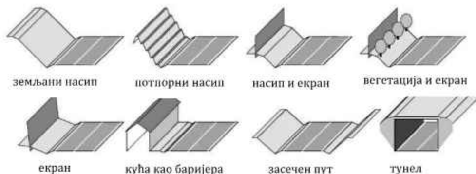
Слика 3.3. Различити типови рефлексионих баријера [44]
