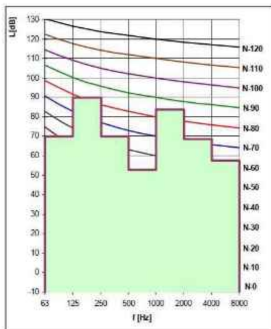
Слика 2.24. Нормативне криве (N-криве) [1].
