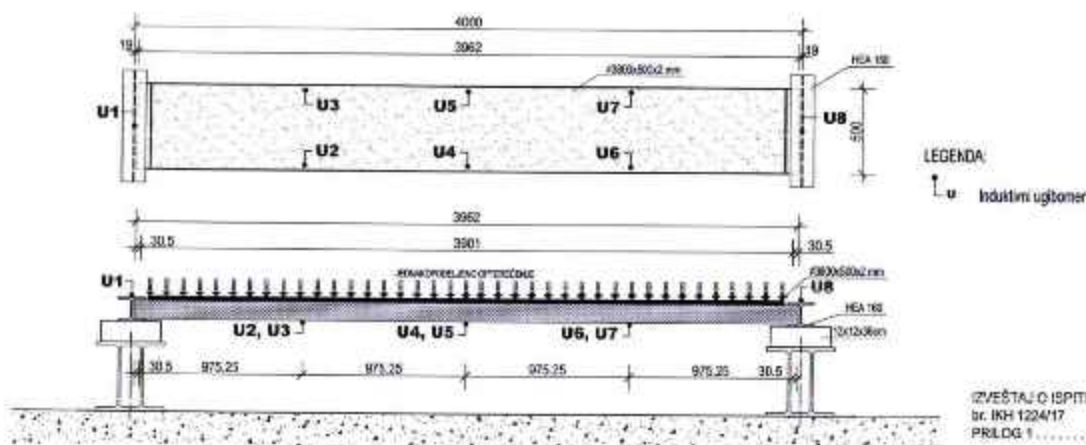
Слика 5.31. Диспозиција испитивања панела за смањење саобраћајне буке на утицај ветра
