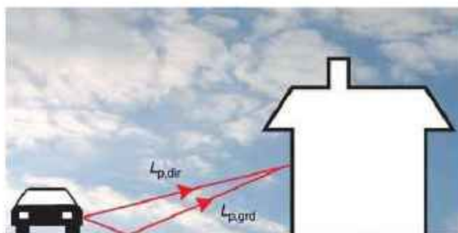
Слика 2.7. Пут неометаног преноса звука [24]
