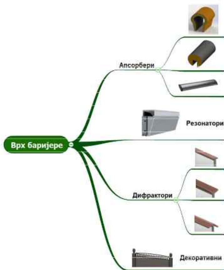
Слика 4.10 Модули врхова баријере
