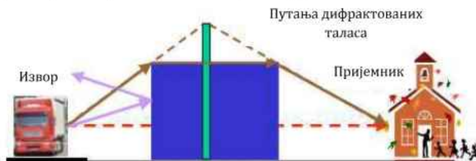
Слика 2.19. Ефекат дебљине баријере [1]
