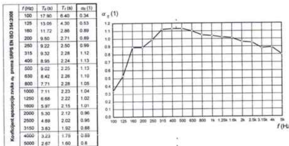
Слика 5.26. Измерене вредности коефицијента апсорпције звука \alpha_0 .
