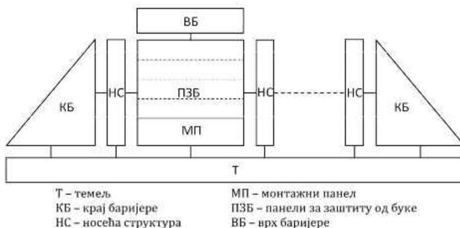
Слика 4.12 Шема поступка конфигурисања модуларне звучне баријере
