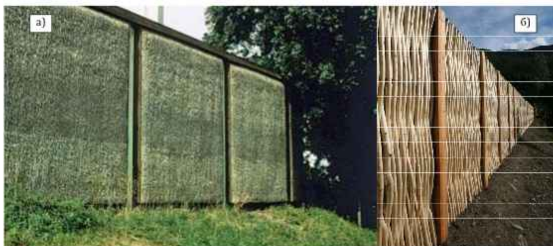
Слика 3.73. Пример баријере од: а) трске [24] и б) плетеног прућа [70]
