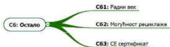
Слика 7.25. Поткритеријумске функције критеријума C6
