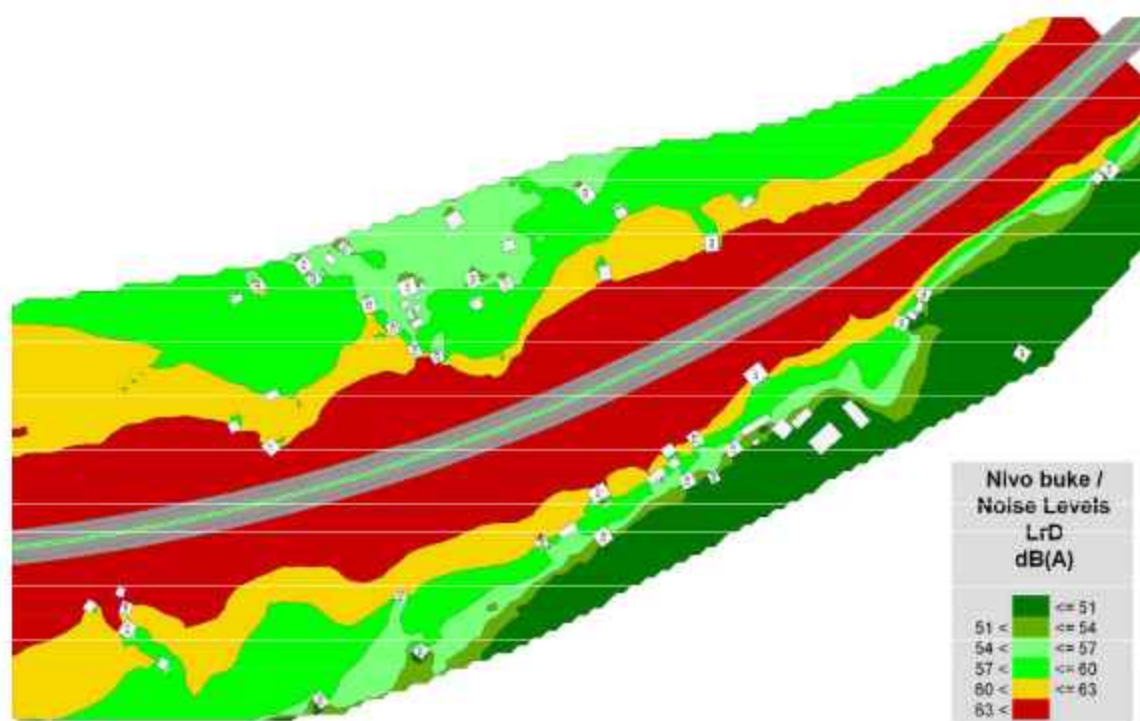
Слика 7.2. Локалитет СТРУПИНА - Карта буке дању, референтно стање [158]
